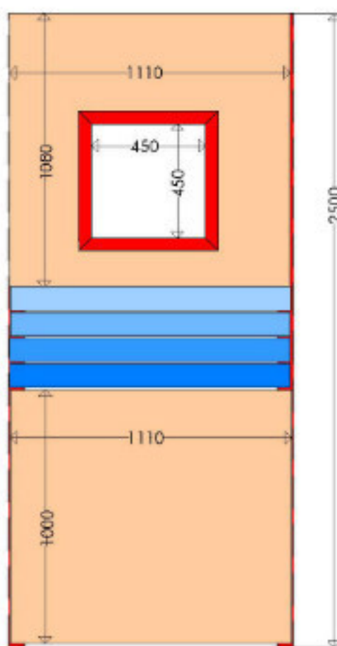
Stirnseite
