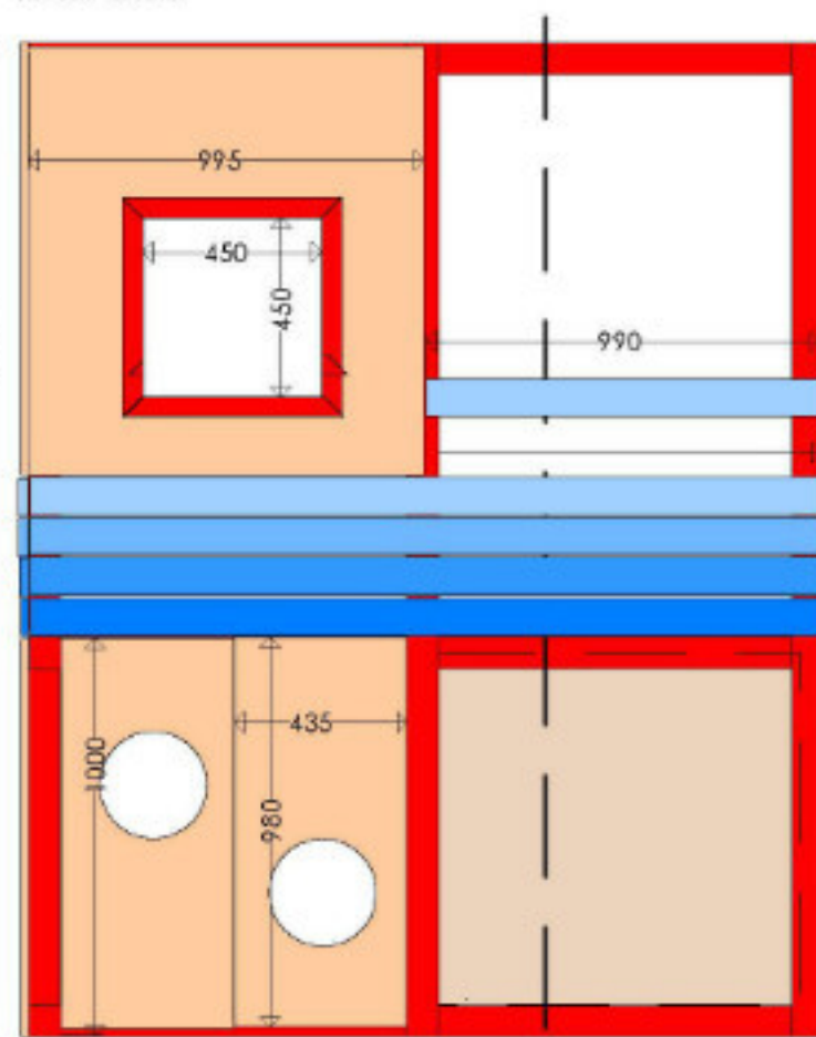
Raumseite
